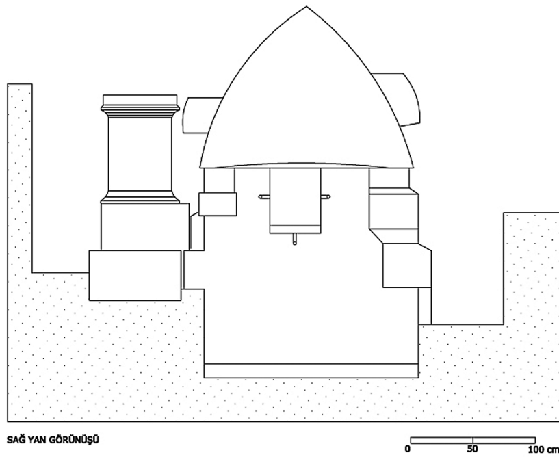
Abb. 19. Die Zeichnung der Grabanlage.
