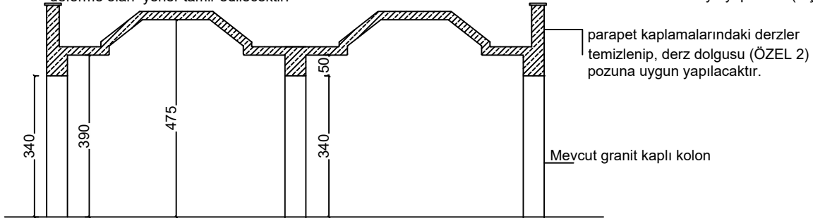
A-A KESİT
