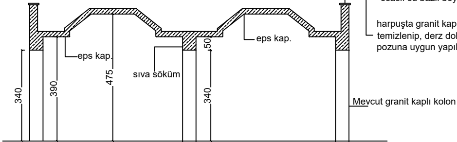
A-A KESİT
