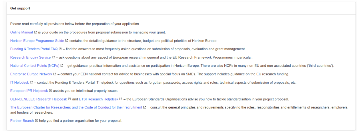
Şekil 14 — Destek bölümü
