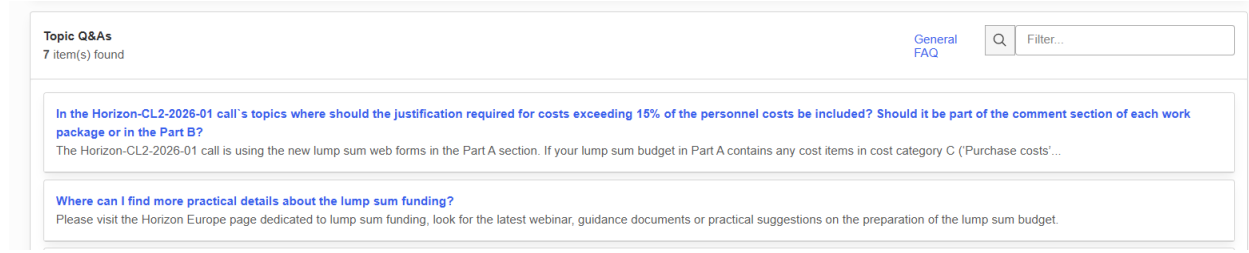
Şekil 13 — Soru-Cevap bölümü
